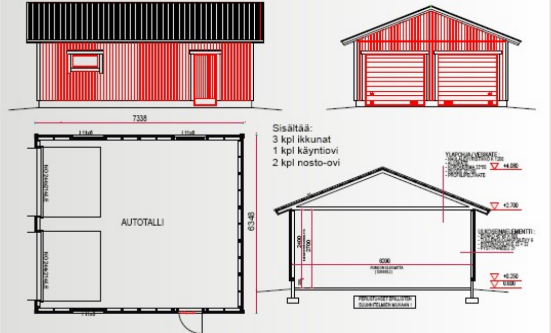
AT 3 Autotalli (7,34x6,35)m. Kerrosale 46,6 m 2 . Huoneistoala 42 m 2 . Sisäkorkeus 2,70m. Tilavuus 140 m 3
