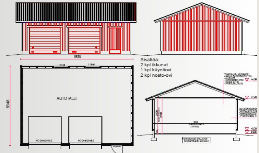
AT 4 Autotalli (8,54x6,35)m. Kerrosale 54,2 m 2 . Huoneistoala 49,2 m 2 . Sisäkorkeus 2,70m. Tilavuus 160 m 3
