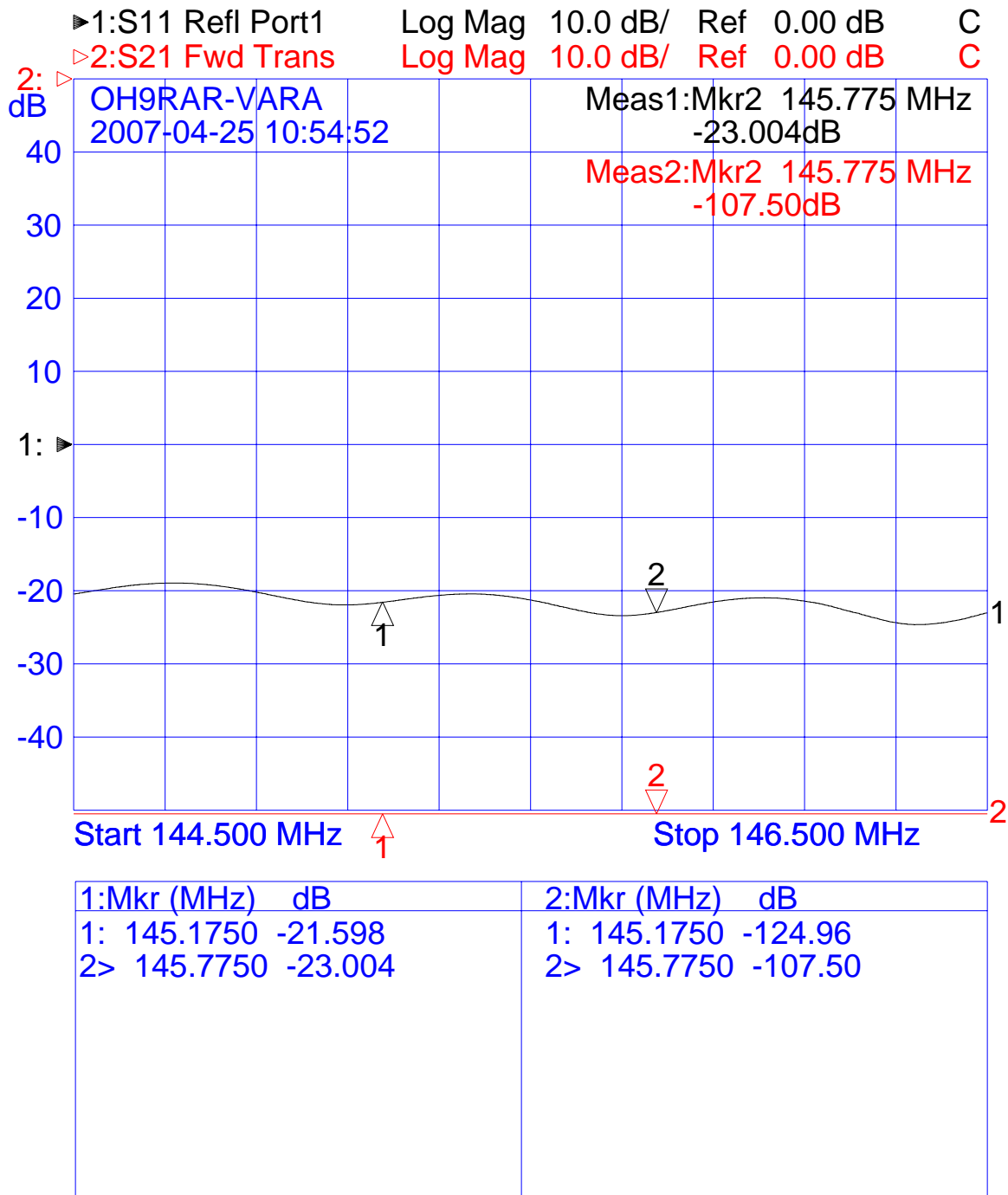
Kuva 5. Heijastusvaimennus antennilinjasta. 145.775 MHz ja SWR on 1.15
