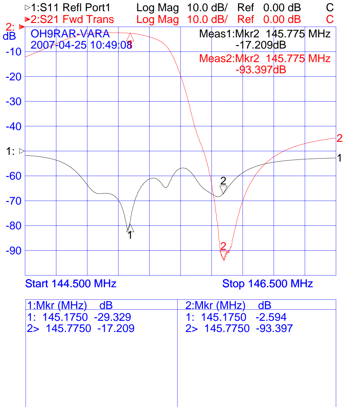
Kuva 1. ANT-portista RX-porttiin. TX-portti sovitettu
