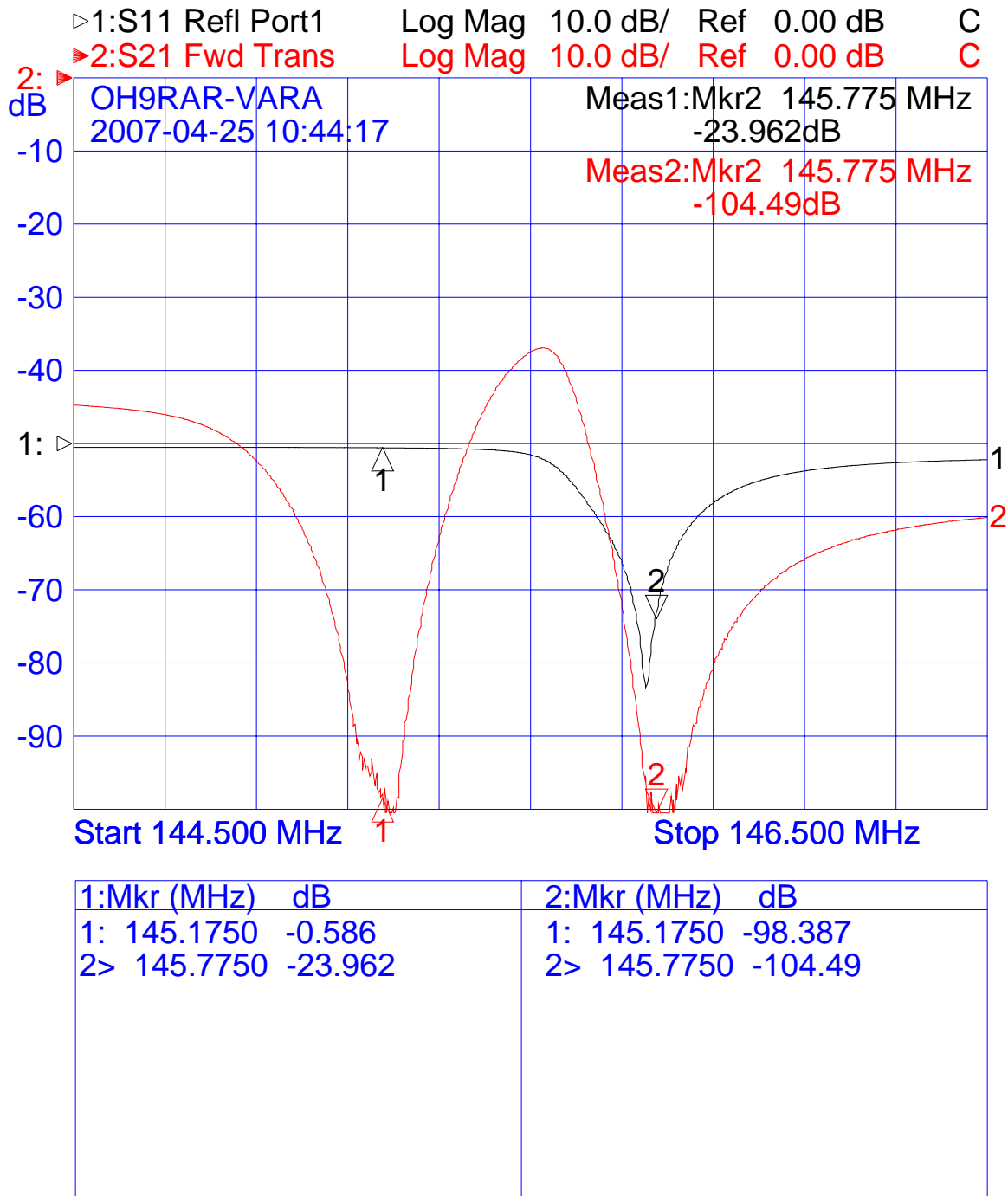
Kuva 3. TX-portista RX-porttiin. ANT-portti sovitettu
